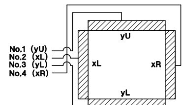
Touch Panel Pin-assign (タッチパネル ピンアサイン)
